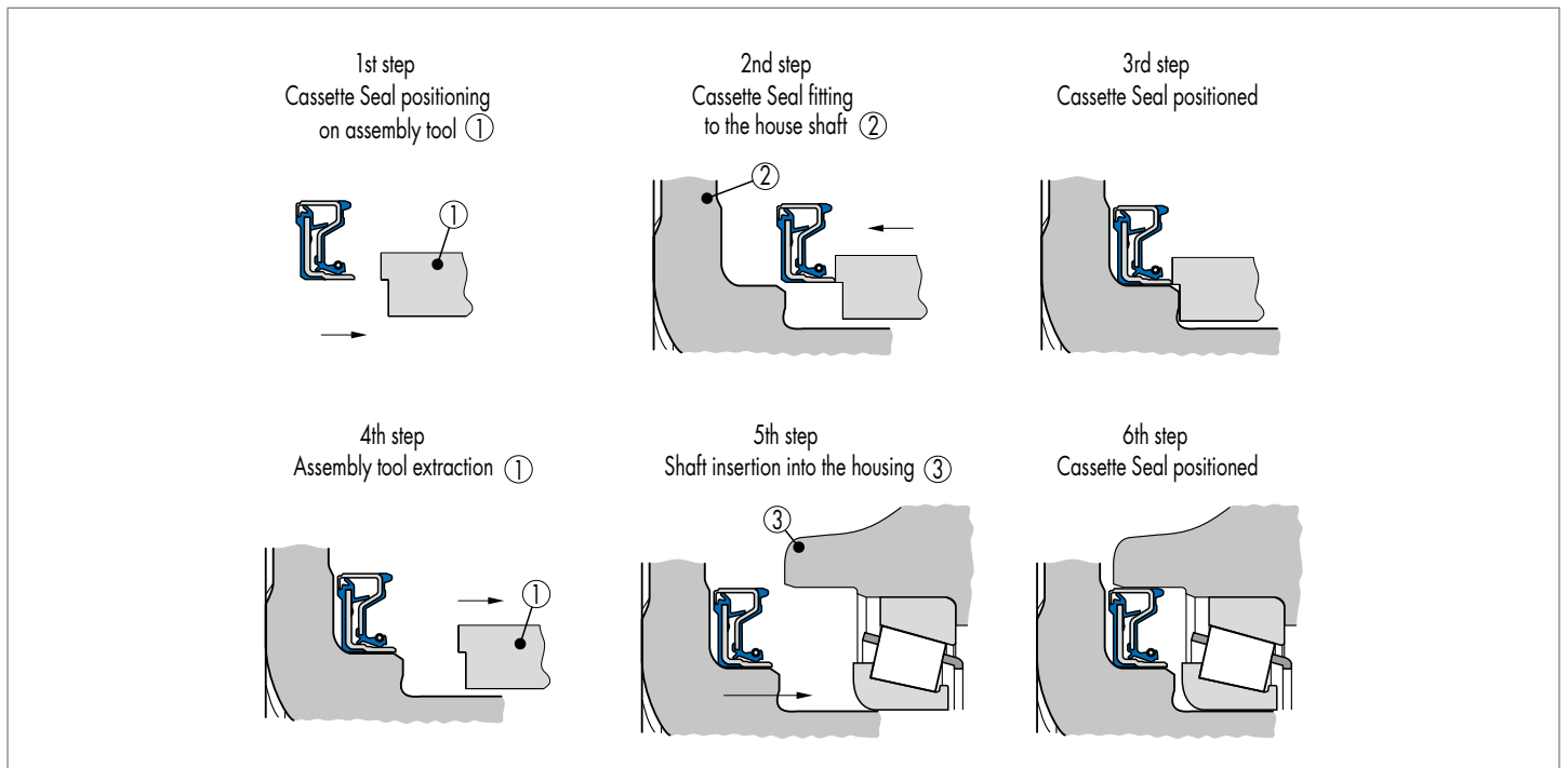
Fig. 20 Installation of Simmering Cassette Seal – Case D ("First on the shaft") / Montage d'une bague Simmering Cassette Seal – Cas D ("d'abord sur l'arbre") / Montaje de Simmering Cassette Seal – caso D ("Primero sobre el eje") / Montagem de anel retentor Cassette Seal – Tipo D ("Primeiro eixo")
