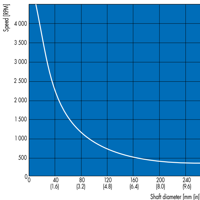
Fig. 4 Permissible speed of Simmerring in rotating housings and fixed shafts. If limits are exceeded, please consult us! / Vitesses admissibles pour alésage tournant et arbre fixe. Si les limites sont dépassées, veuillez consulter nos services ! / Máxima velocidad para retenes con alojamientos rotativos y ejes fijos. Si se sobrepasan los límites ¡Consúltenos! / Velocidade permitida de Simmerrings em alojamentos rotativas e eixos fixos. Se excedidos os limites, por favor consulte-nos!
