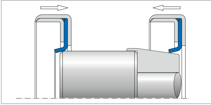
Fig. 14 Installing a Simmerring with sealing lip made of PTFE / Montage d'une bague Simmerring avec lèvre d'étanchéité en PTFE / Montaje de un retén Simmerring con labio de sellado de PTFE / Montagem de retentor Simmerring com lábio de vedação em PTFE
