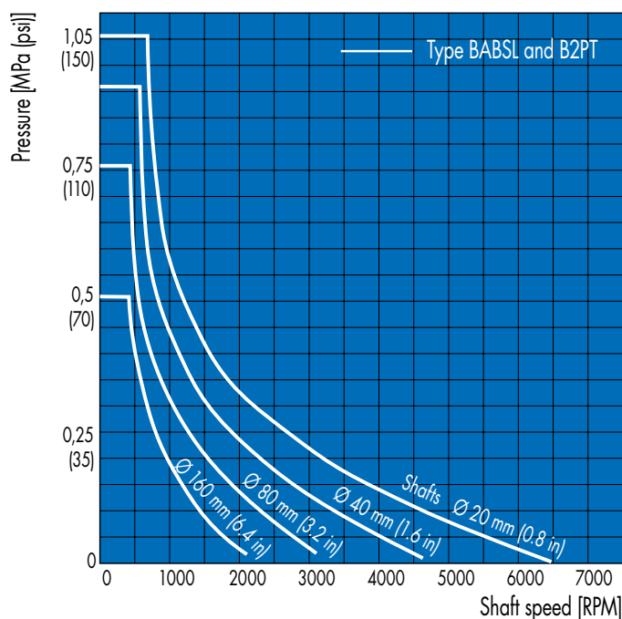
Fig. 2 Permissible pressure in the unit for Simmerring (Type BABSL and B2PT) / Pression admissible dans le mécanisme pour les bagues d'étanchéité Simmerring (type BABSL et B2PT) / Presión admisible en el grupo para retenes Simmerring (Forma constructiva BABSL y B2PT) / Pressão admissível no subgrupo para anéis retentores (modelo construtivo BABSL e B2PT)
