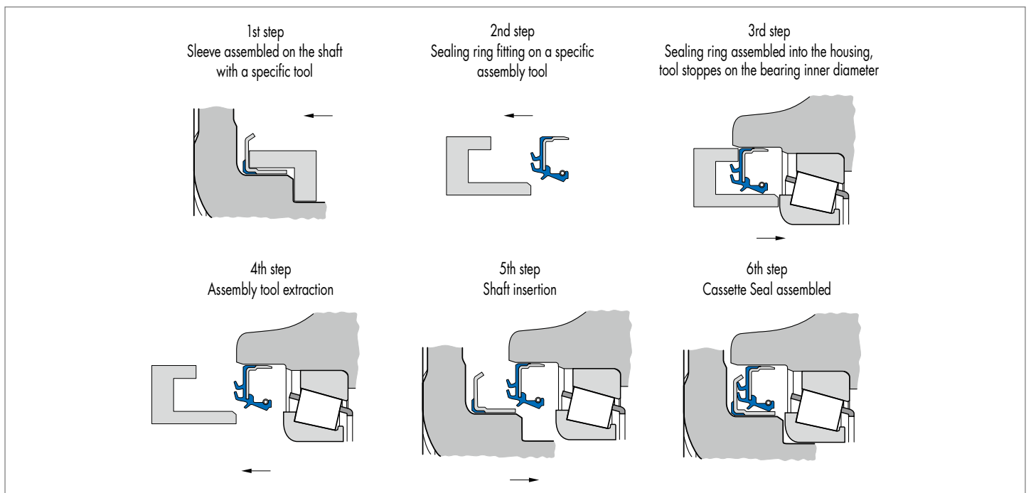
Fig. 21 Installation Case E ("2-Step-Assembly") for special types in split execution / Montage d'une bague Simmering Cassette Seal – Cas E ("2 étapes d'assemblage") pour des formes de construction spéciales dans l'exécution divisée / Montaje de Simmering Cassette Seal – caso E ("Asamblea en 2 pasos") para diseños especiales en la ejecución de división / Montagem de anel retentor Cassette Seal – Tipo E ("Montagem em dois passos") para projetos especiais em execução dividida
